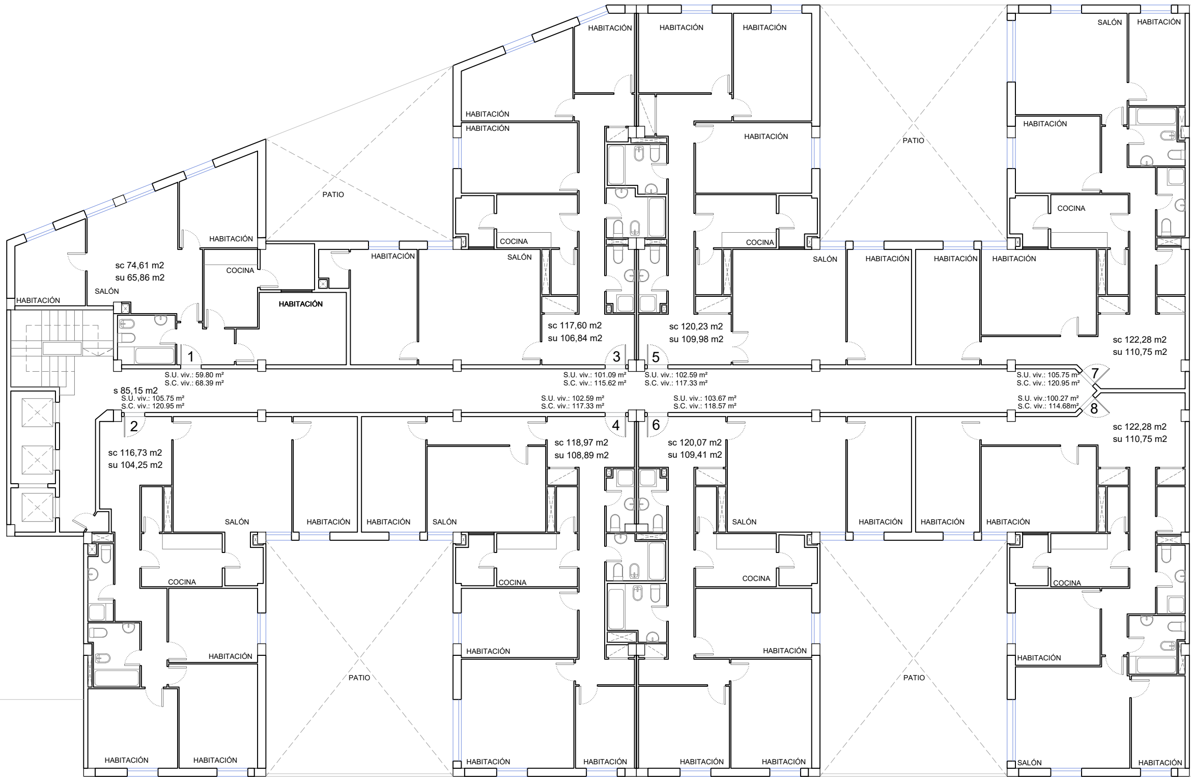
PLANTA TIPO_VIVIENDAS
